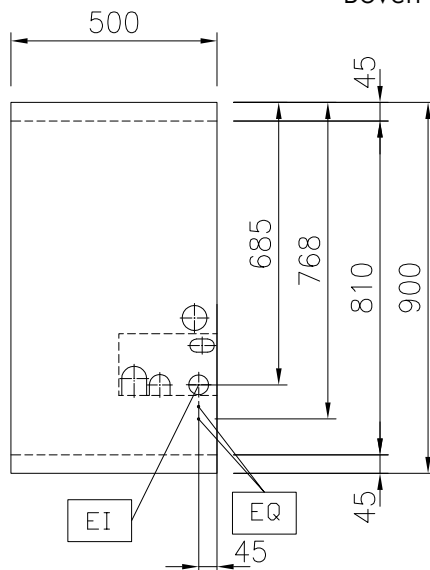
Boven aanzicht
